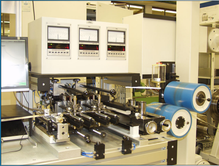
Zwei Banddickenmeßgeräte, ein Bandbreitenmeßgerät Two Strip Thickness Gauges, Strip Width Gauge
